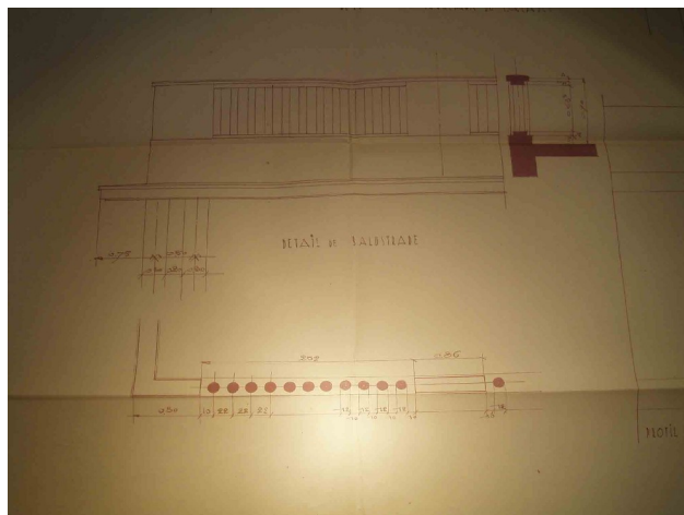
Garde-corps, détail, dessin d'Ali Tur, 1931, ANOM
